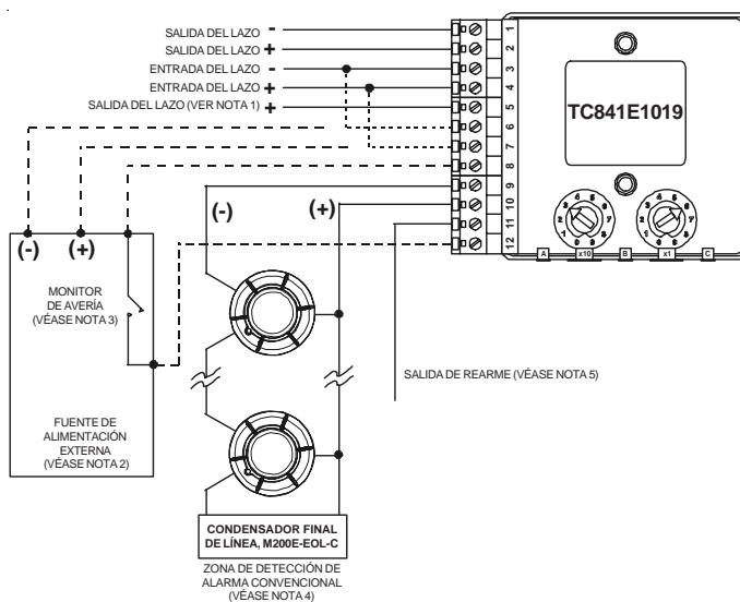
FIGURA 3: MÓDULO MONITOR PARA ZONAS CONVENCIONALES TC841E1019
